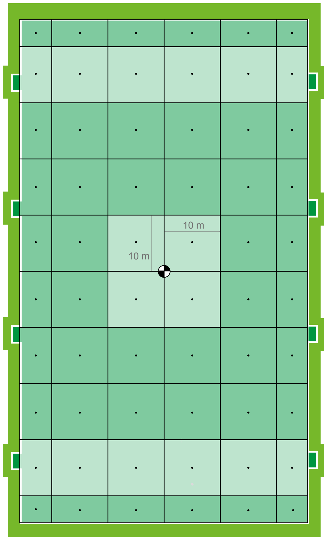
Schéma maillage éclairage
