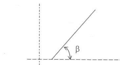
Figure E. 5.1.2.2.1. Angle \beta d'une paroi de tranchée non blindée
