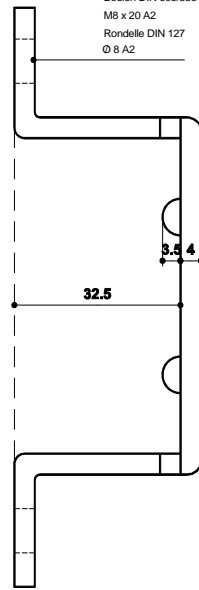
1/2 Bride droite
