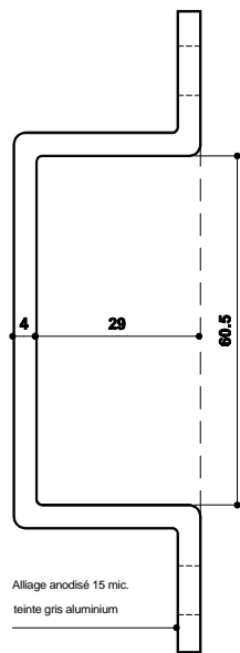
1/2 Bride gauche
