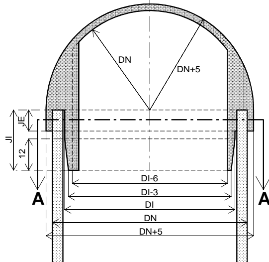
COUPE B-B
